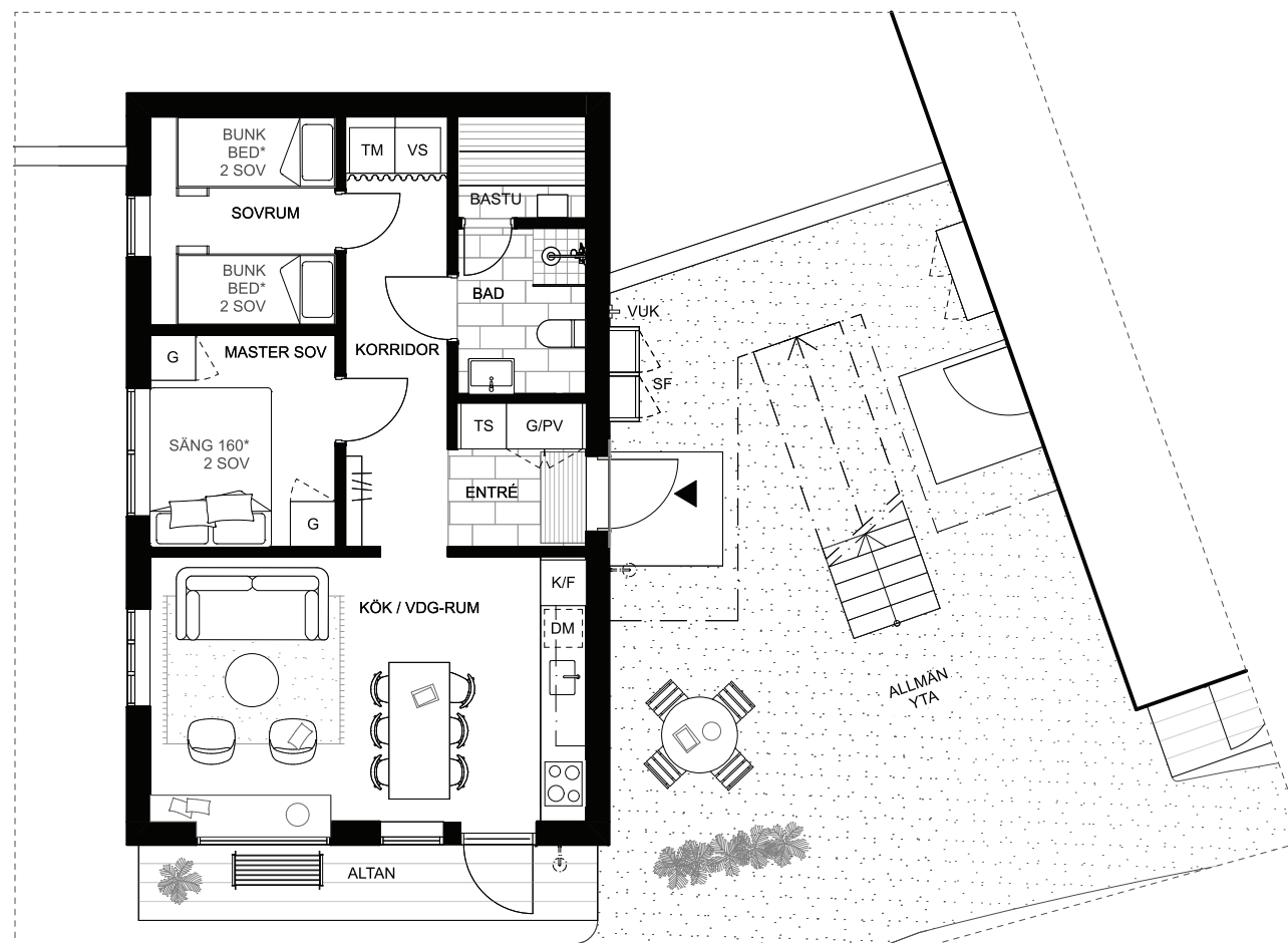
PLAN -1, SUTERRÄNGVÅNING
