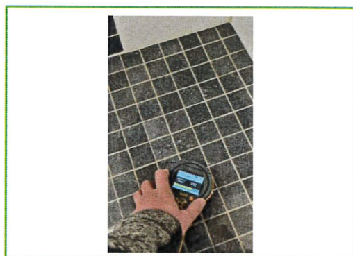
Bild 4: Inga förhöjda fuktvärden uppmättes i badrum.
