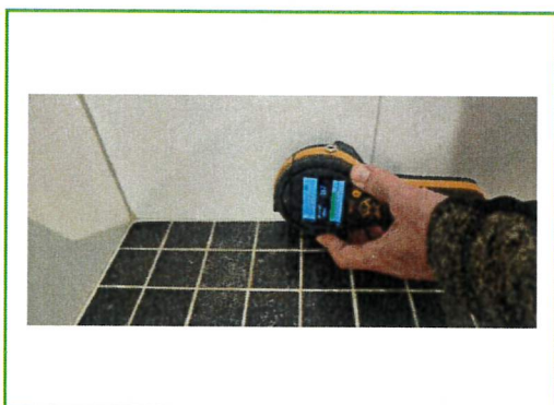
Bild 5: Inga förhöjda fuktvärden uppmättes i badrum.
