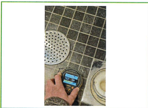
Bild 3: Inga förhöjda fuktvärden uppmättes i badrum.
